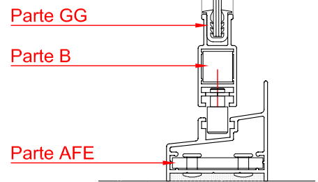
CORTE 3-3
