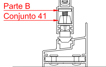
CORTE 1-1
