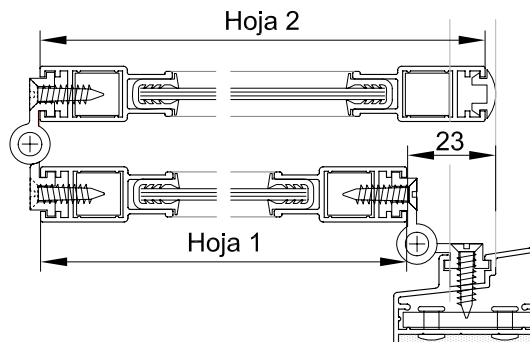
Dimensiones de corte de perfiles
