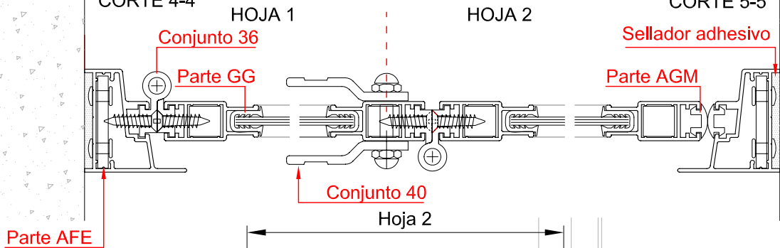
CORTE 4-4
