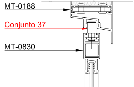
CORTE 3-3
